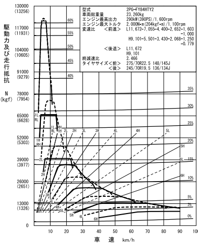
⑮ FY84HTY2 (OD12段ShiftPilot+2.466、標準)
