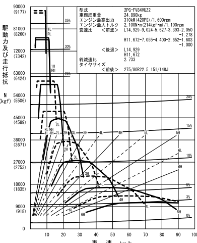
㉒ FV84VUZ2 (直結12段ShiftPilot+2.733、標準)
