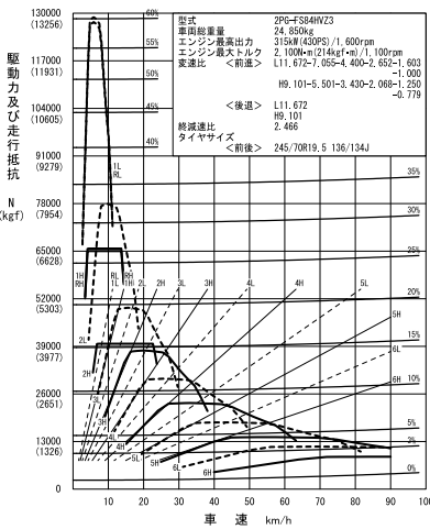
⑬ FS84HVZ3 (OD12段ShiftPilot+2.466、標準)
