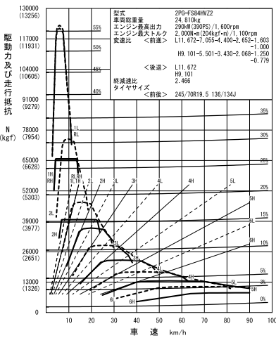
⑫ FS84HVZ2 (OD12段ShiftPilot+2.466、標準)
