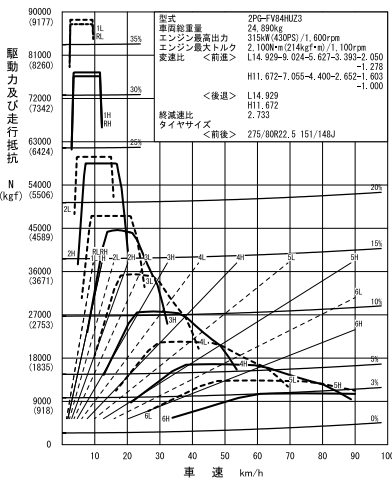
㉑ FV84HUZ3 (直結12段ShiftPilot+2.733、標準)
