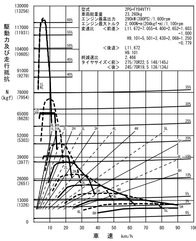
⑯ FY84VTY1 (OD12段ShiftPilot+2.466、標準)
