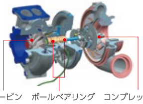
タービン ボールベアリング コンプレッサ
