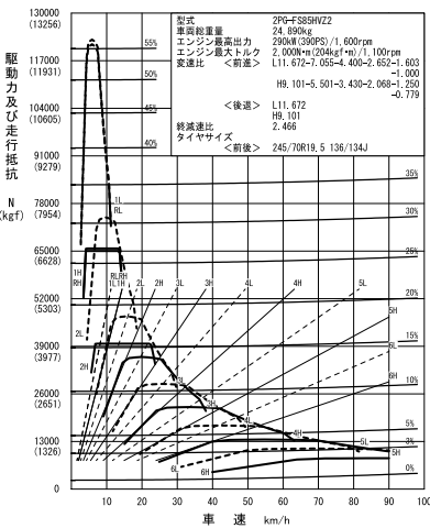
⑲ FS85HVZ2 (OD12段ShiftPilot+2.466、標準)
