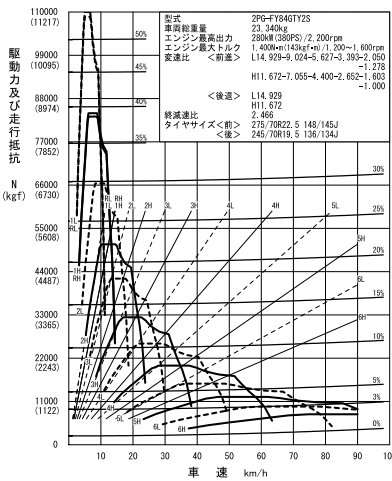
⑭ FY84GTY2S (直結12段ShiftPilot+2.466、標準)
