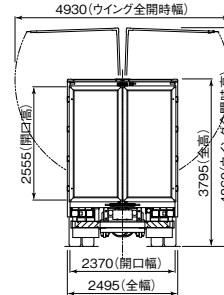
●パブコ製ボデーサイズ(mm)
