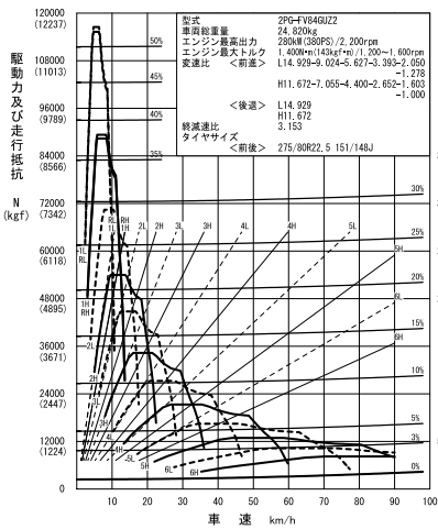
⑳ FV84GUZ2 (直結12段ShiftPilot+3.153、標準)
