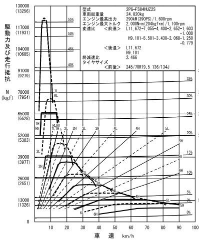
⑪ FS84HUZ2S (OD12段ShiftPilot+2.466、標準)
