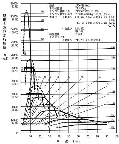
⑰ FS84VVZ1 (OD12段ShiftPilot+2.466、標準)
