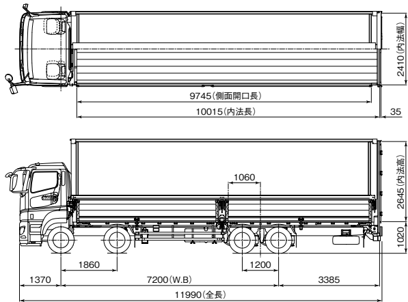
■2PG-FS84GUZ2S* (ショートキャブ、標準仕様)
