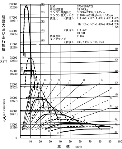
⑱ FS84VVZ2 (OD12段ShiftPilot+2.466、標準)
